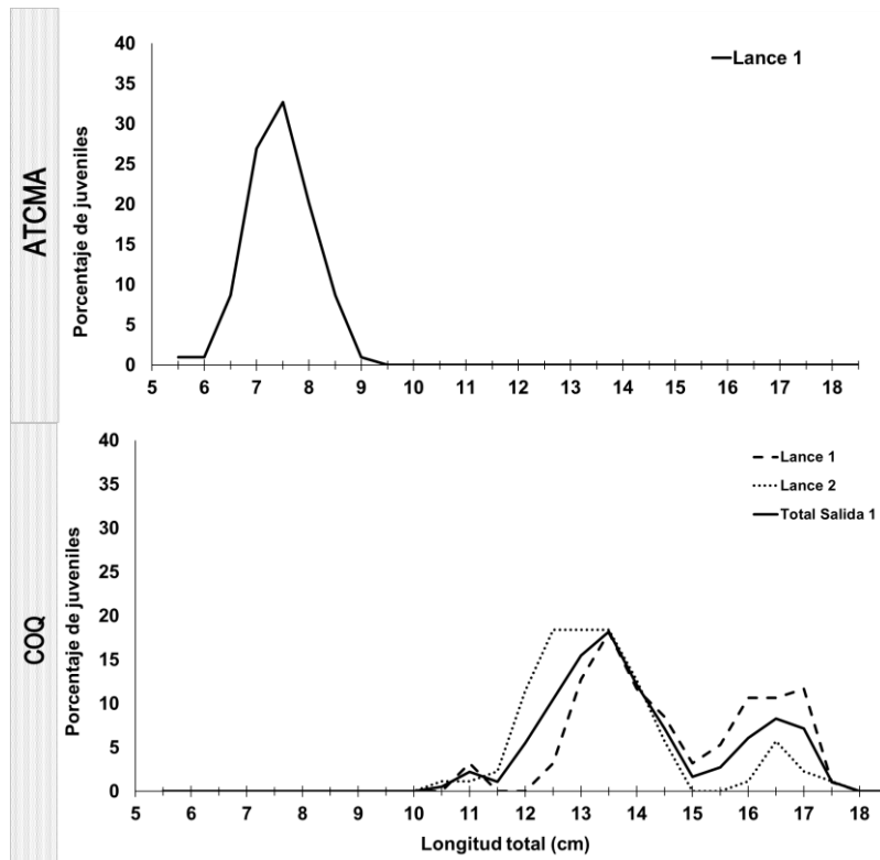
Figura 1. Estructura de talla (cm) de los lances muestreados de la PINV, regiones de Atacama y Coquimbo
