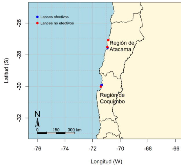
Figura 2. Posición geográfica de los viajes muestreados de anchoveta, flota artesanal, zona centro norte.
